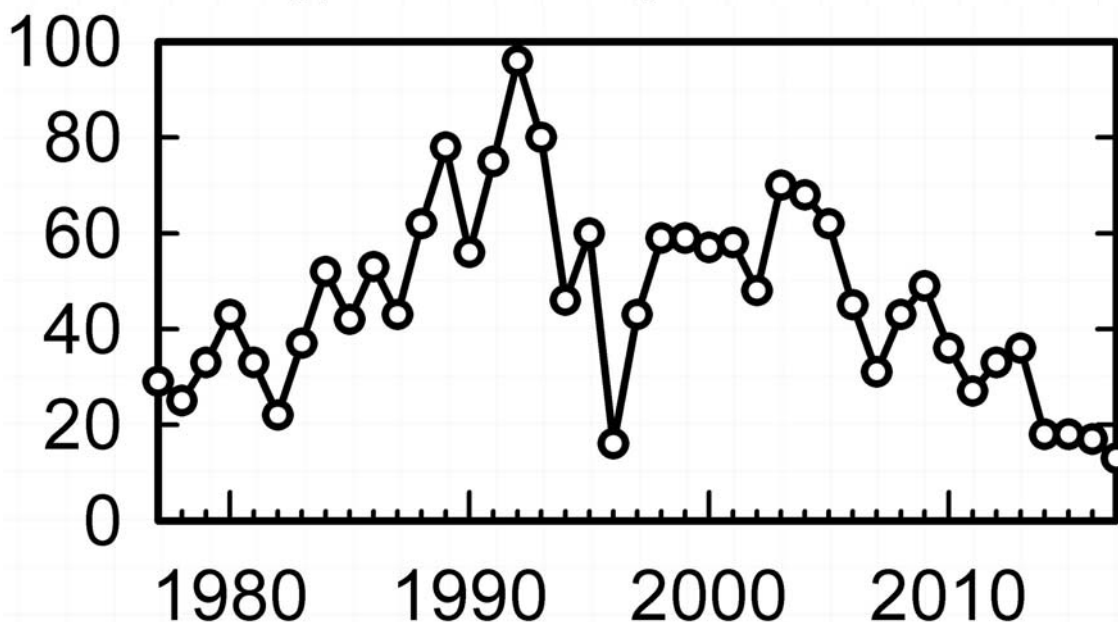
Fig 2: Ynglepar på Elleore Breeding pairs at Elleore
