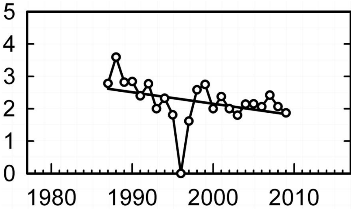
Fig 12: Kuldstørrelse i juli syd for Eskilsø Broodsize in July south of Eskilsø
