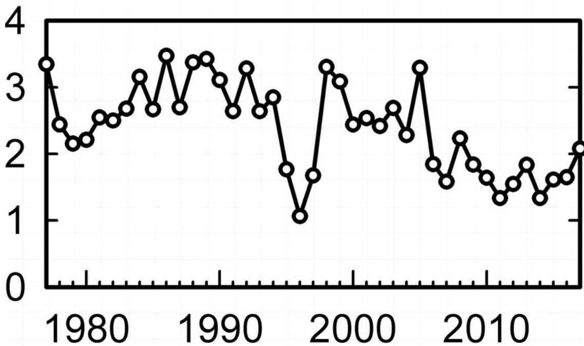
Fig 8: Unger per rede på Elleore Cygnets per nest at Elleore
