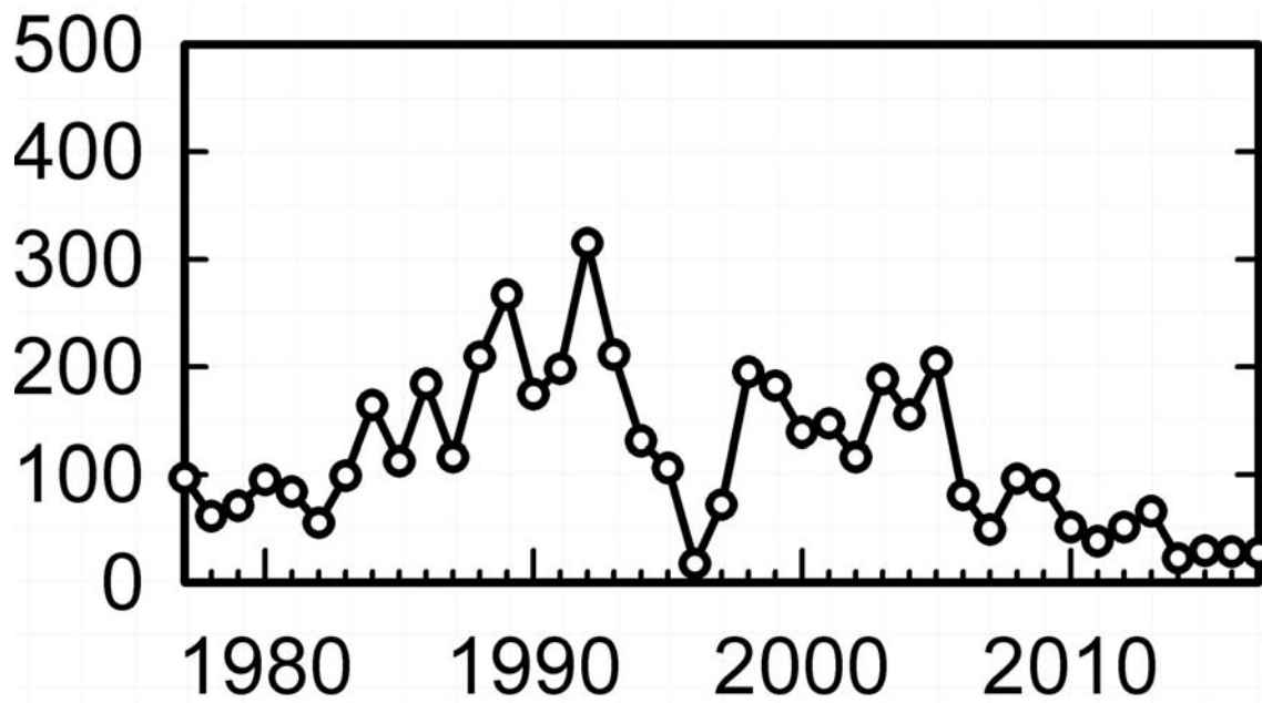
Fig 7: Unger på Elleore Cygnets at Elleore
