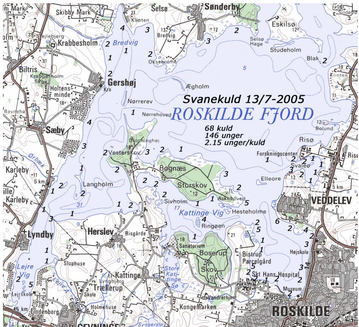
Fig 14: Eksempel på kuldernes fordeling (Juli 2005). Tallene er kuld størrelser Example of the distribution of broods (July 2005). The numbers are brood sizes
