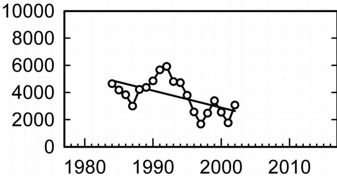
Fig 16: Oktober bestand i Roskilde Fjord October population in Roskilde Fjord
