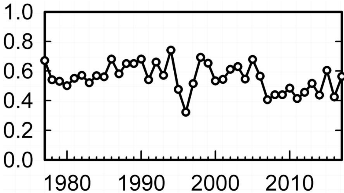
Fig 9: Unger per æg på Elleore Cygnets per egg at Elleore
