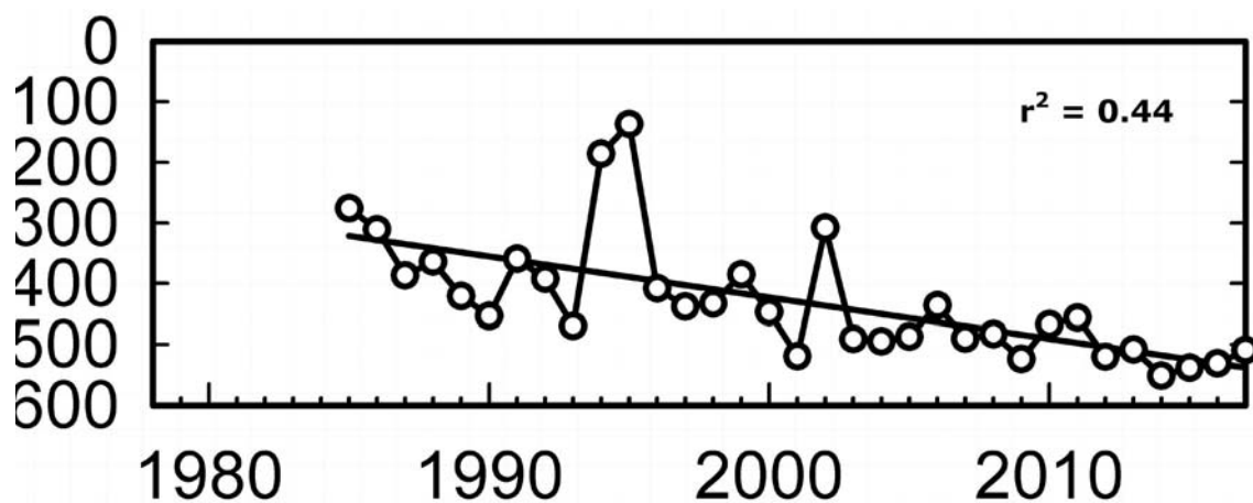
Fig17. Sommersigtddybde i Lejre Vig (cm) Summer Secchi depth in Lejre Vig (cm)
